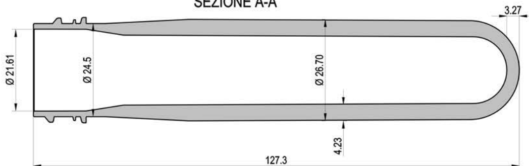
SEZIONE A-A
